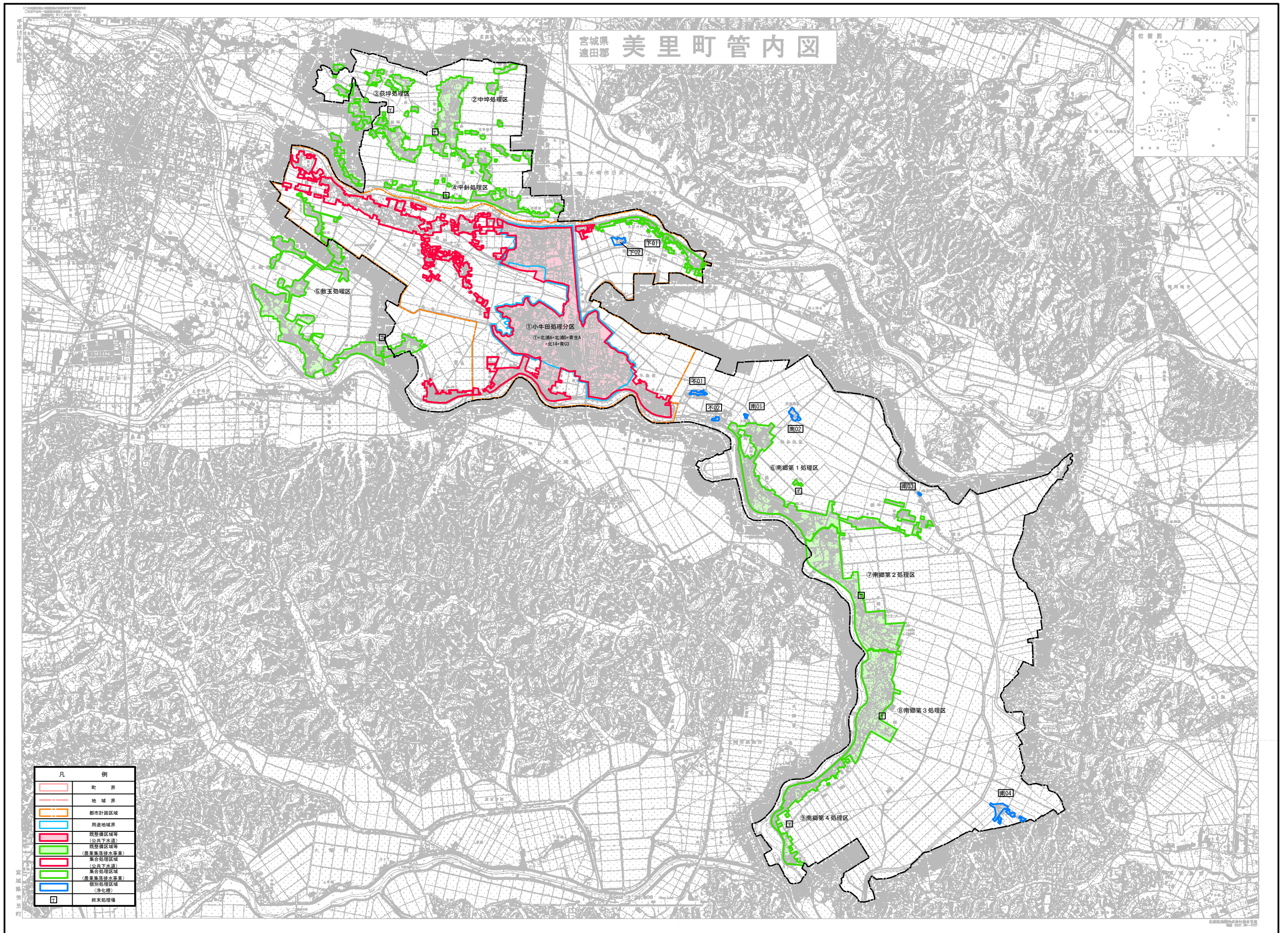
検討図9 経済性を基にした集合処理区域同士の接続検討 判定結果
