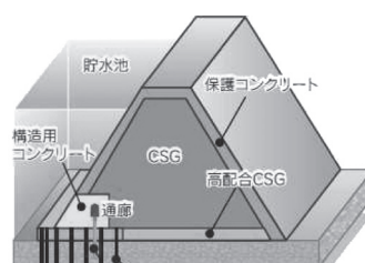
▲鳴瀬川ダムの構造
