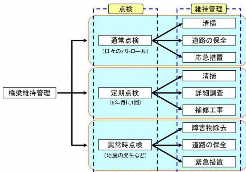
図2. 橋梁の点検および維持管理の体系
