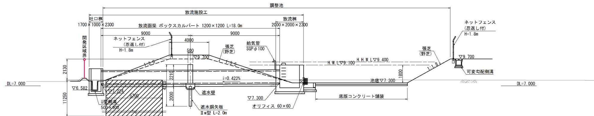
B-B' 断面図
