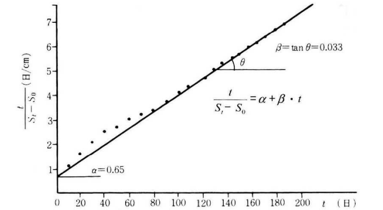
参図 7-2 双曲線法におけるパラメータの推定の例
