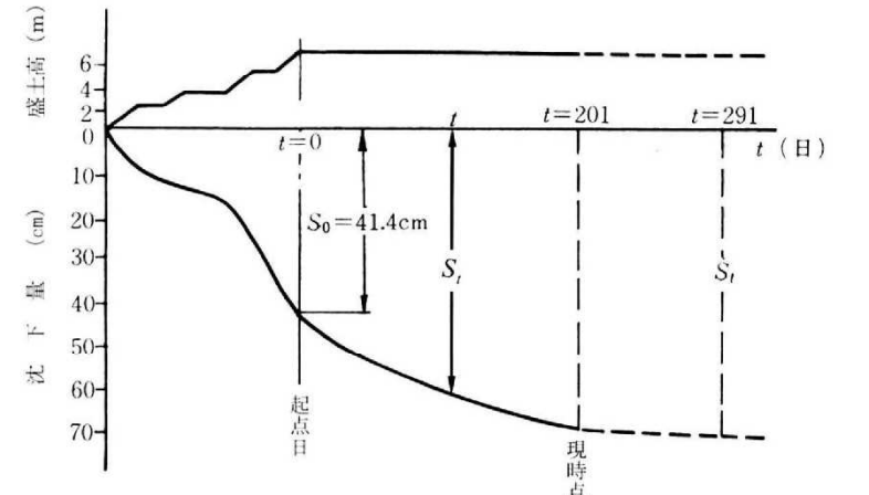
参図 7-1 実測沈下曲線と双曲線法による予測の例
