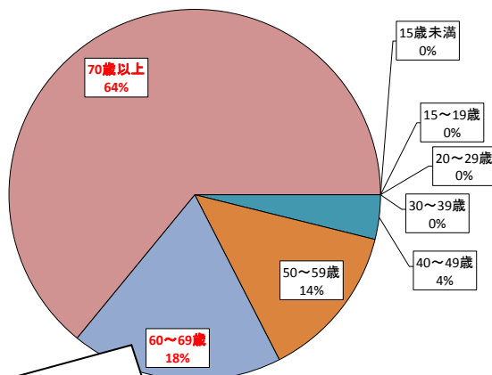
死亡事故の年齢別割合（宮城県：H15～24）
