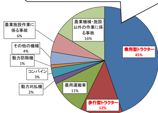
死亡事故の農業機械別割合（宮城県：H15～24）
