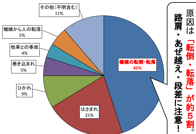
機械作業に係る要因別割合（宮城県：H15～24）
